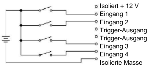
Abbildung 31: Anschluss mit einer Fremdspannungsquelle
