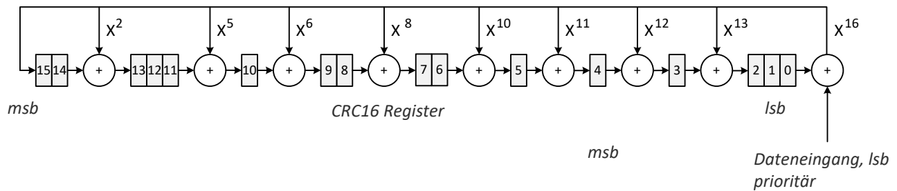
Abbildung 59: Schieberegisterstruktur für dieses Polynom
