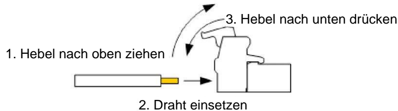
Abbildung 37: Draht einsetzen
