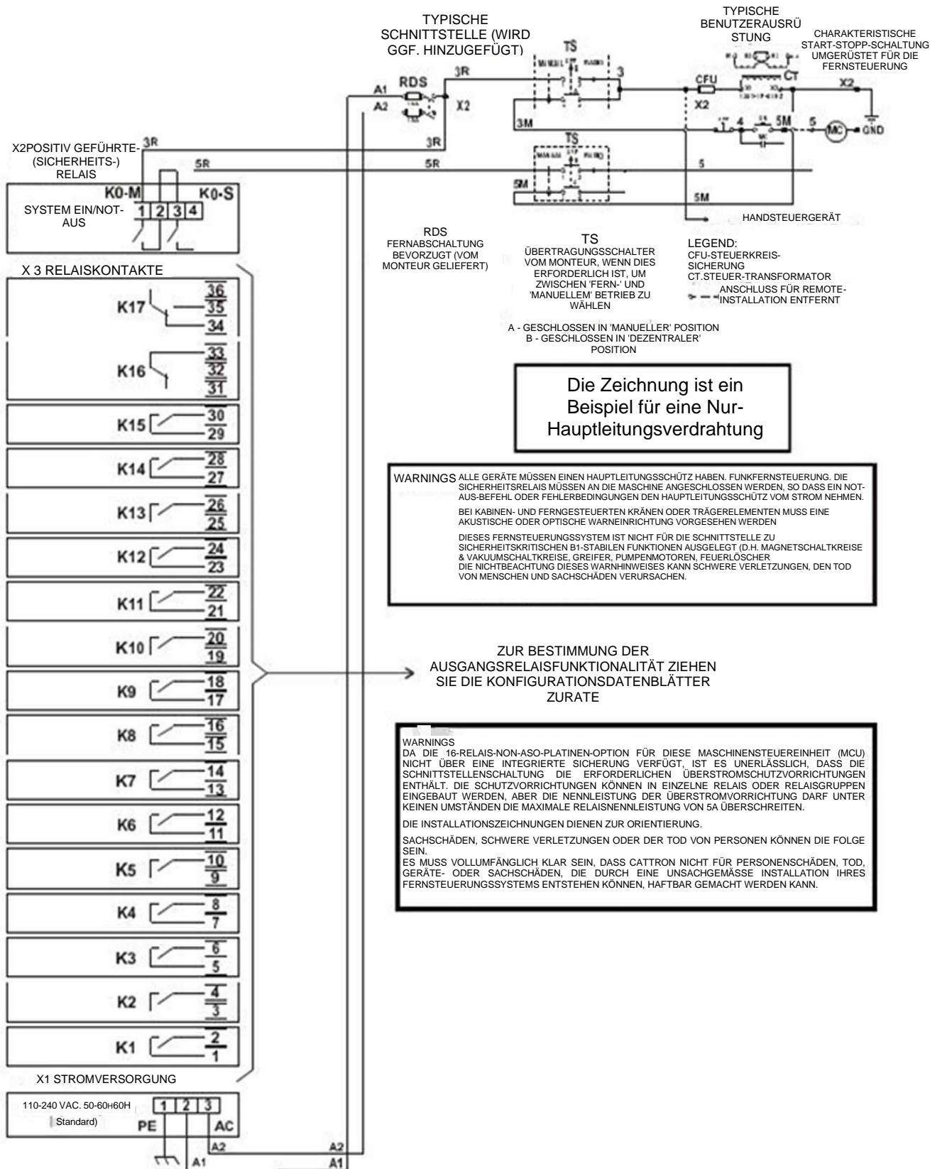
Abbildung 41: Beispielszeichnung Hauptleitung
