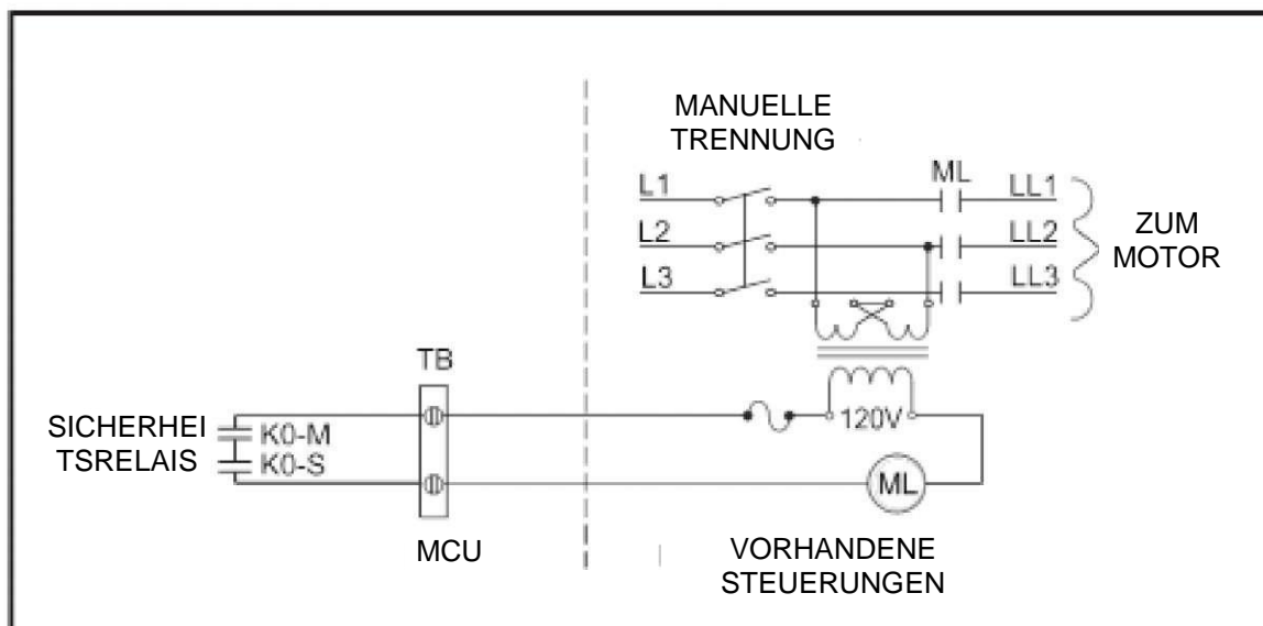
Abbildung 43: Sicherheitsrelaiskontaktverdrahtung
