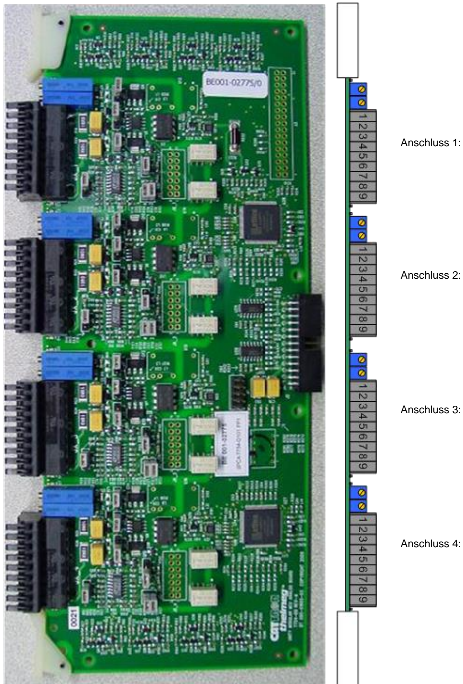
Abbildung 15: Analoge Platine
