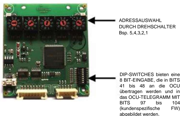
Abbildung 45: IR Controllerplatine
