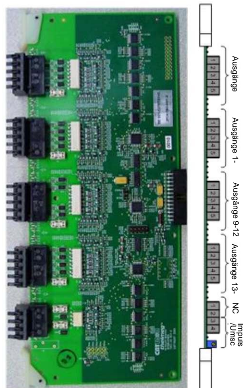
Abbildung 28: Digitale Ausgangsplatine
