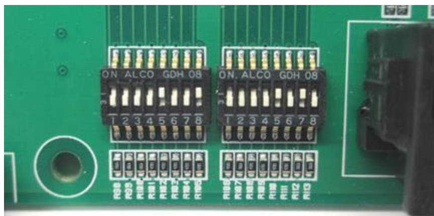
Abbildung 23: 16 Positionen Dip-Schalter
