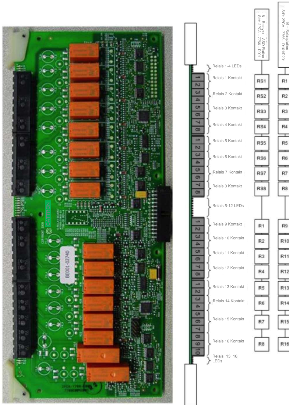
Abbildung 12: Relaiskarte
