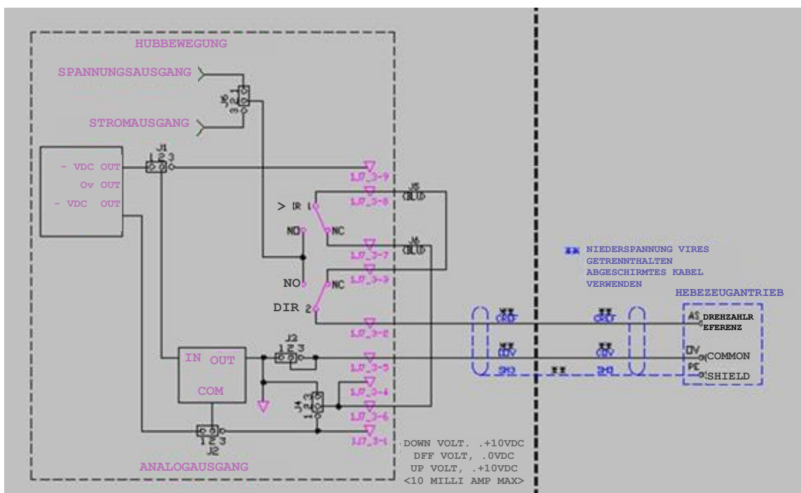
Abbildung 16: Analogausgang Schaltbild
