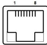
Abbildung 13: RJ45-Klinkensteckeranschluss
