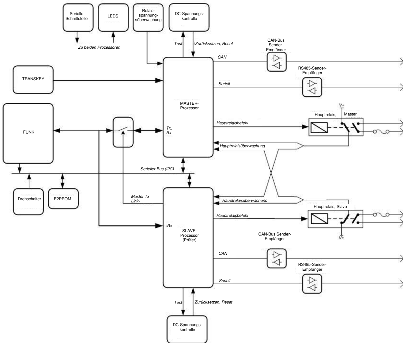
Abbildung 2: Blockdiagramm
