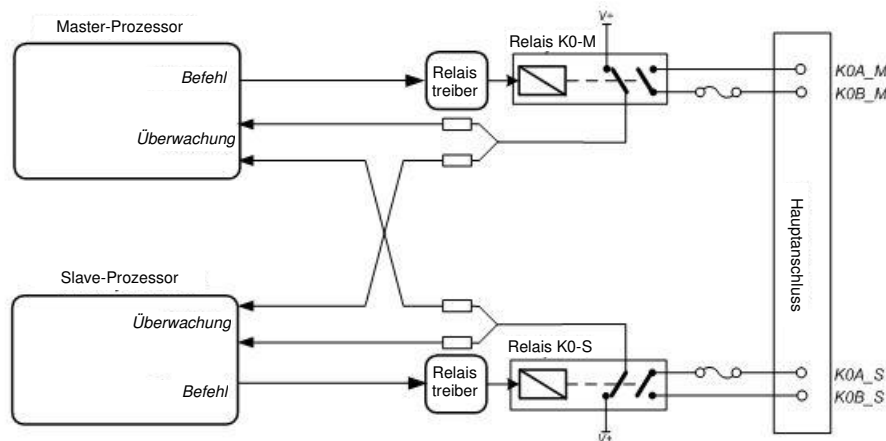
Abbildung 6: Sicherheitsrelais-Schnittstelle Blockdiagramm
